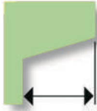
Standard (angle 15°) Profondeur d'onglet réglable jusqu'à 18mm
